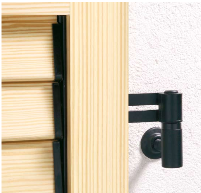
La bandella a scomparsa su cardine a muro.
